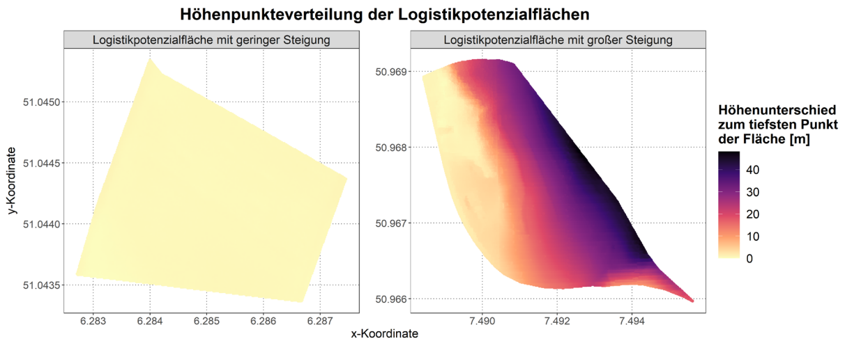
Abbildung 77: beispielhafte Gegenüberstellung der Höhenpunkteverteilung zweier Logistikpotenzialflächen
