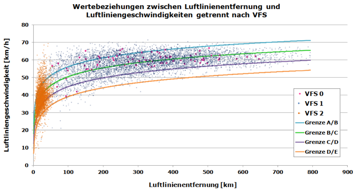
Abbildung 40: SAQ-Kurven im Straßengüterverkehr (Klemmer 2016)
