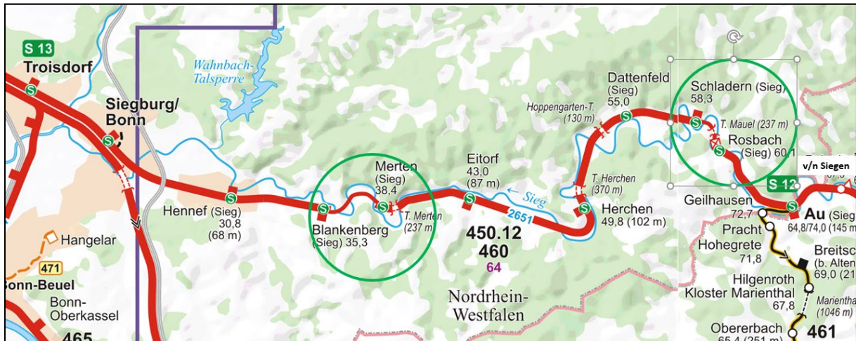
Abbildung 123: Zweigleisiger Ausbau der Siegstrecke (Quelle: Verlag Schweers + Wall 2020)
