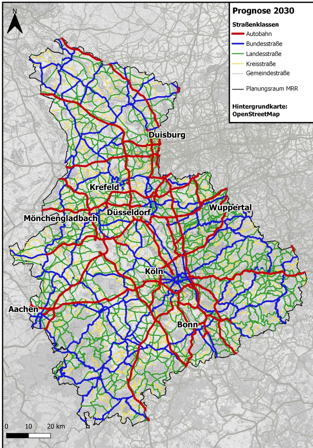
Abbildung 102: Untersuchungsrelevantes Straßennetz der Prognose 2030 im Planungsraum
