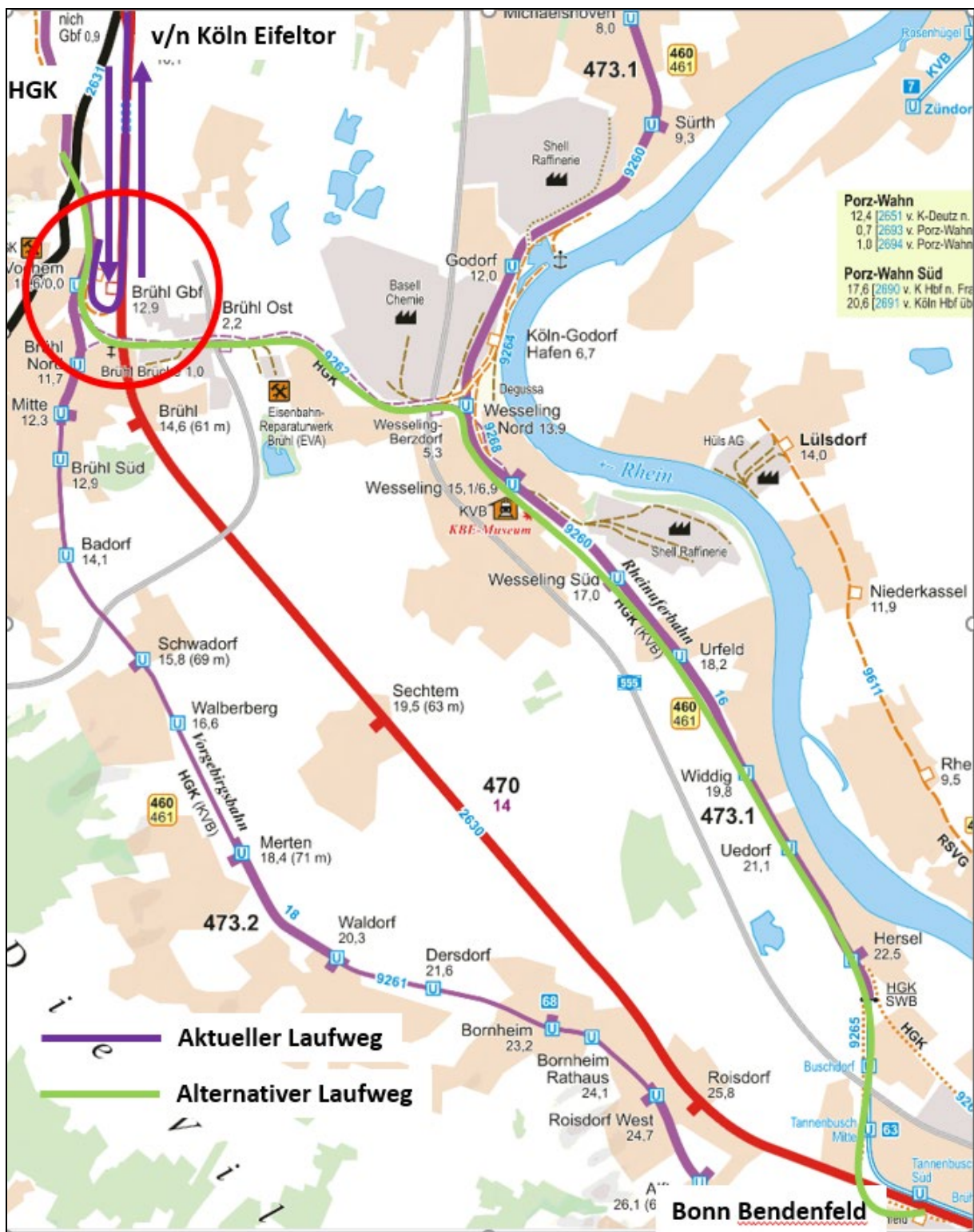
Abbildung 121: Einbindung des HGK-Netzes ab Bonn Bendenfeld (Quelle: Verlag Schweers + Wall 2020)
